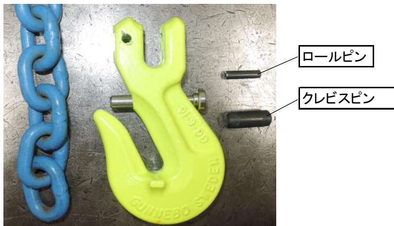
②クレビスピンを挿入する
