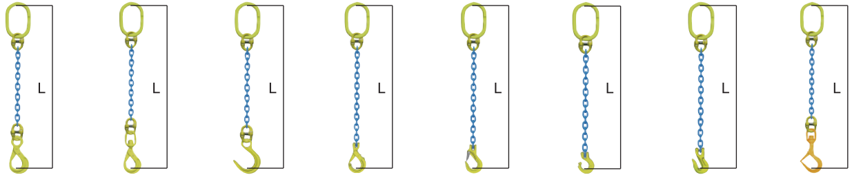
TA1-BK TA1-BKL TA1-OKE TA1-GBK TA1-EGKNA TA1-CL (チョーク・バスケット吊り用) TA1-GGA (チョーク吊り用) TA1-BMS (敷き鉄板吊り用)
